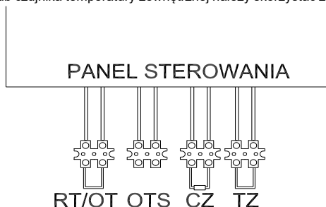
Rys.3.9.1 Płytkę sterownika
