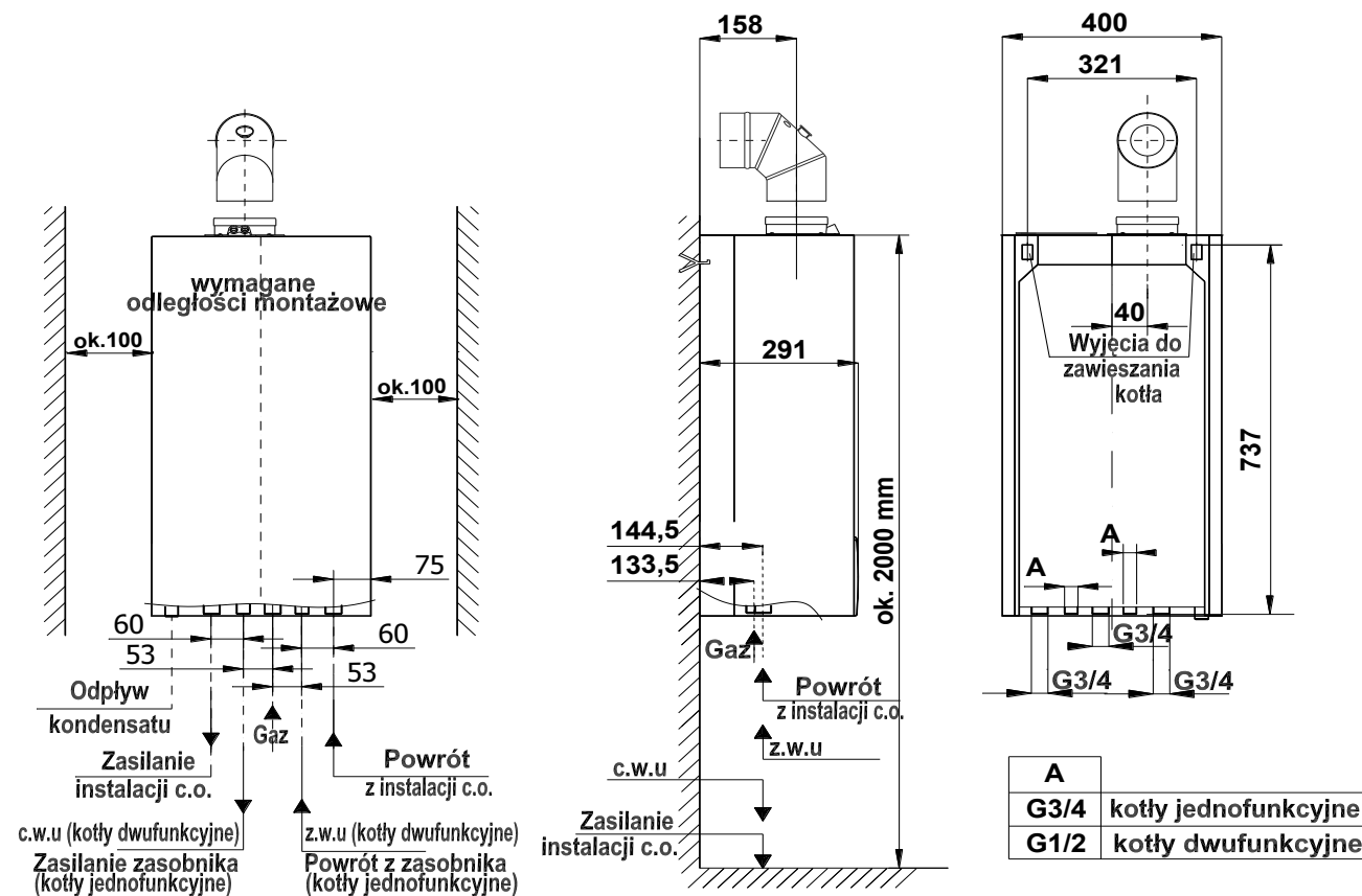
Rys. 3.3.1 Wymiary instalacyjne kotłów ECOCONDENS CRYSTAL II PLUS
