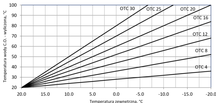
Krzywa grzewcza
